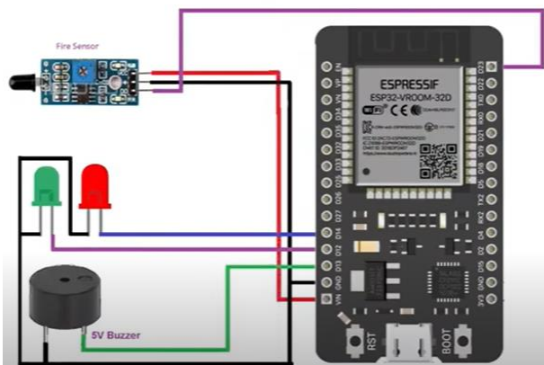
Alur rangkaian sensor api
