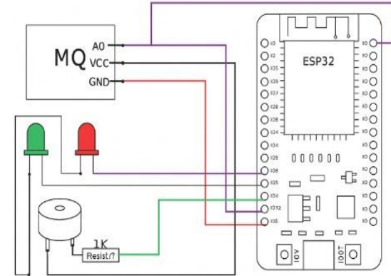
Alur rangkaian sensor asap
